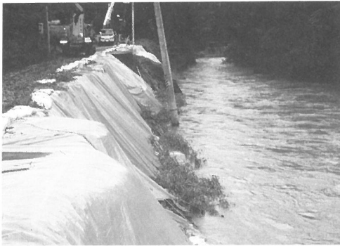
▲高蔵内地区の道路が崩れ水道管が折れる
