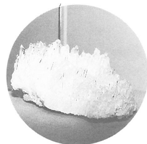
透明水晶の群晶（スイス産）
