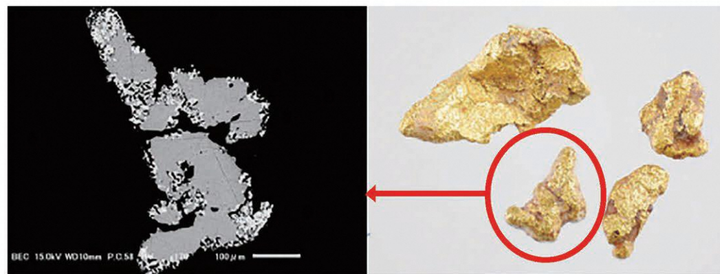
外側の白色部は金の純度が高く 灰色部は銀の含有率が高い(電子像)
