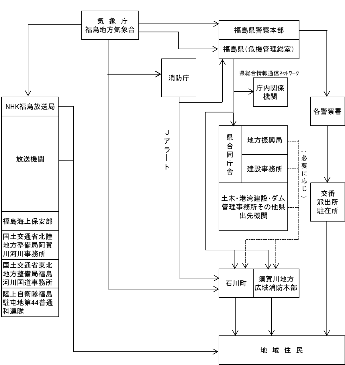
地震情報等伝達系統図
