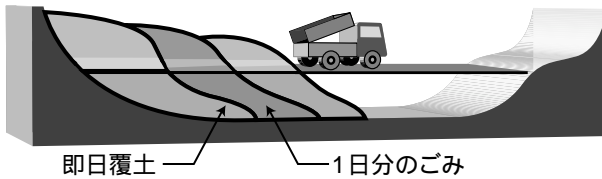
セル工法（略図）
